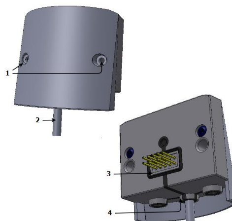
Fig. 6. Structure of the APT-ELF2-USB-1 module
